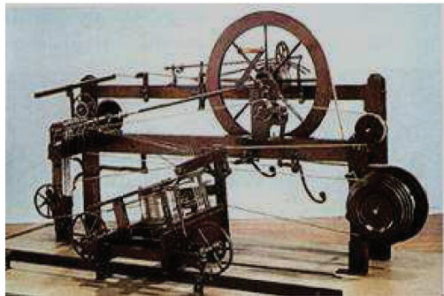
الشَّكل (٥) اخترع صموئيل كرومبتون المِغزَلُ الآليَّ عام ١٧٧٦م، واستخدمه في غزلِ القطن.
