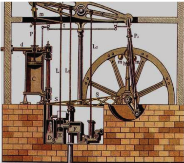
الشَّكل (٦) صنعُ توماس نيوكُمن محركاً بخاريّاً عام ١٧١٢م لاستخراج الفحم.
